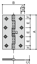
■サイズ表 (単位:mm)
